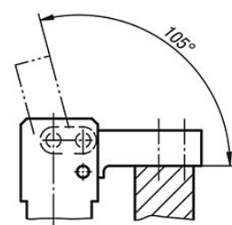
Forme A Force de serrage verticale, angle d'ouverture max. 105 degrés
