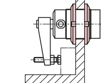
Avec deux écrous à encoche.
