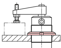
Avec un écrou à encoche par le haut.
