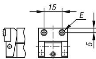
3 inserts carrés en carbure pour le M10
