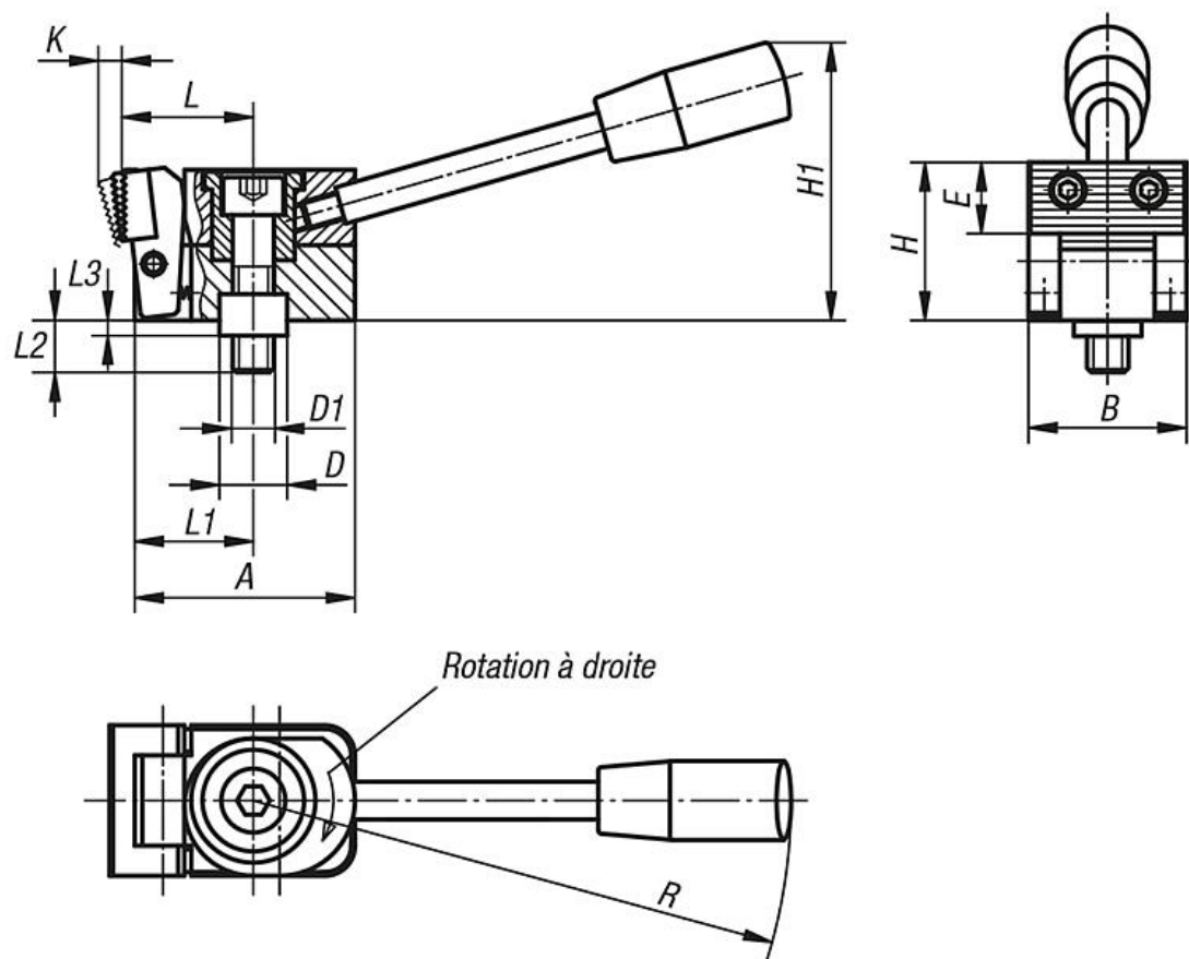
Forme A Mors strié en acier traité
