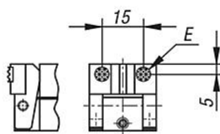
2 inserts carrés en carbure et vé de centrage pour le M10
