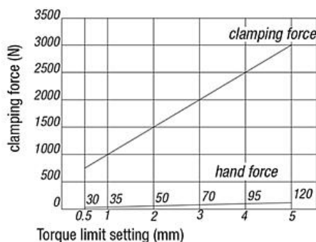
Side Clamps 04565-0500 04565-0501
