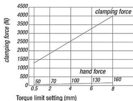
Side Clamps 04565-0800 04565-0801
