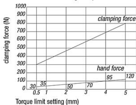
Swing Clamps 04366-...3232
