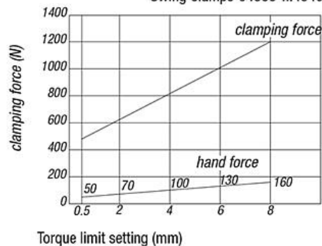
Swing Clamps 04366-...4540
