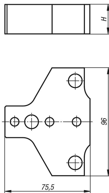
Zvýšení pomocí adaptéru pro pevnou stranu
