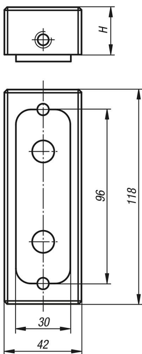
Zvýšení pomocí adaptéru pro pohyblivou stranu
