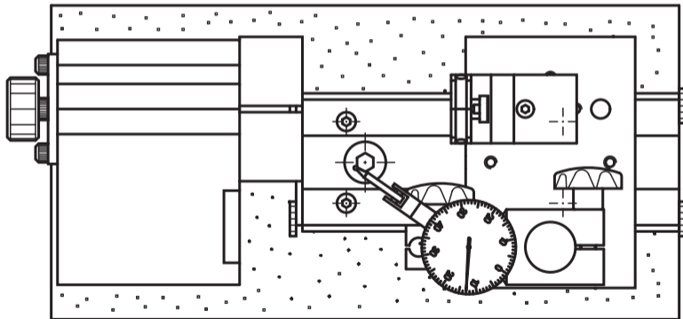
Příklad s prizmou jako opěrné ložisko pro dlouhé díly
