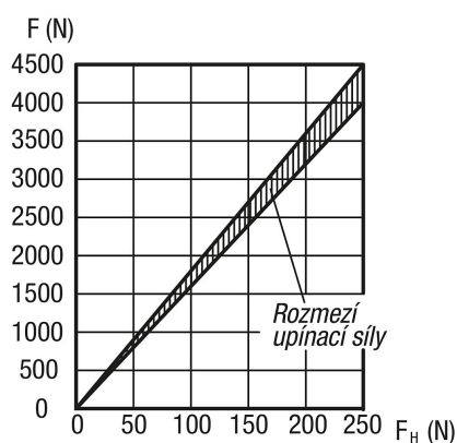
Silový diagram
