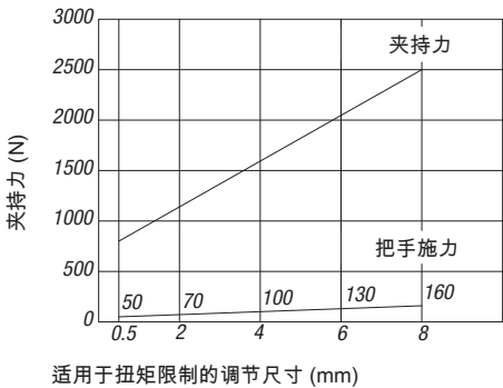
拉紧夹具 04400-4050...
