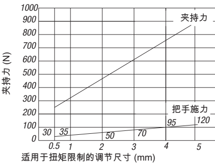
拉紧夹具 04400-3240...
