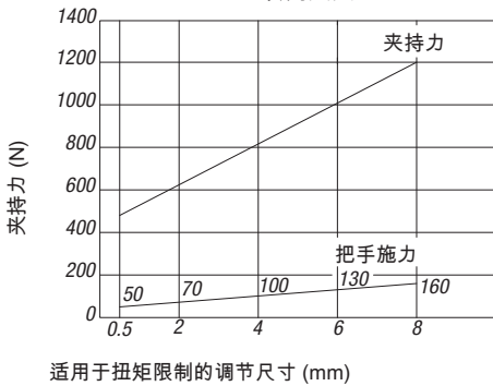
转角夹具 04366-...4540
