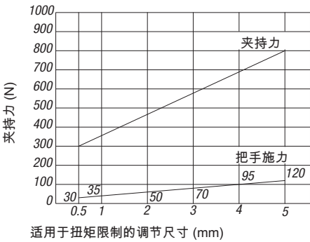
转角夹具 04366-...3232
