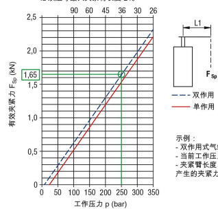
夹紧力示意图
