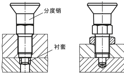
定位 带定位衬套
