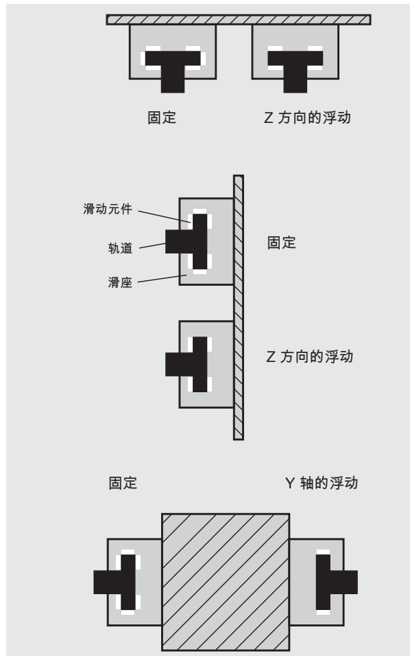
在 Z 轴方向和活动主轴水平安装
