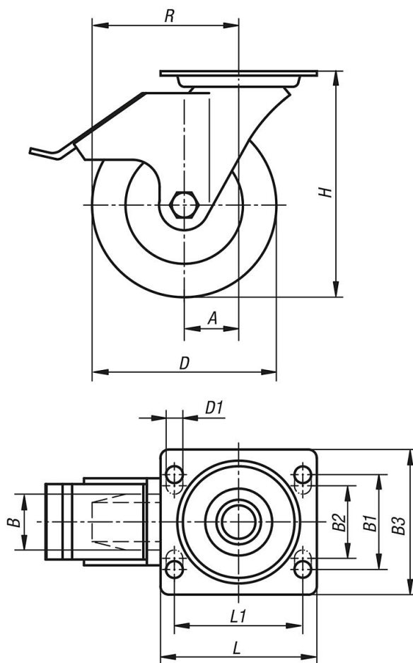
带“stop fix”的 转向轮
