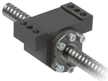
Vis à bille avec écrou à collerette emmanché dans le support
