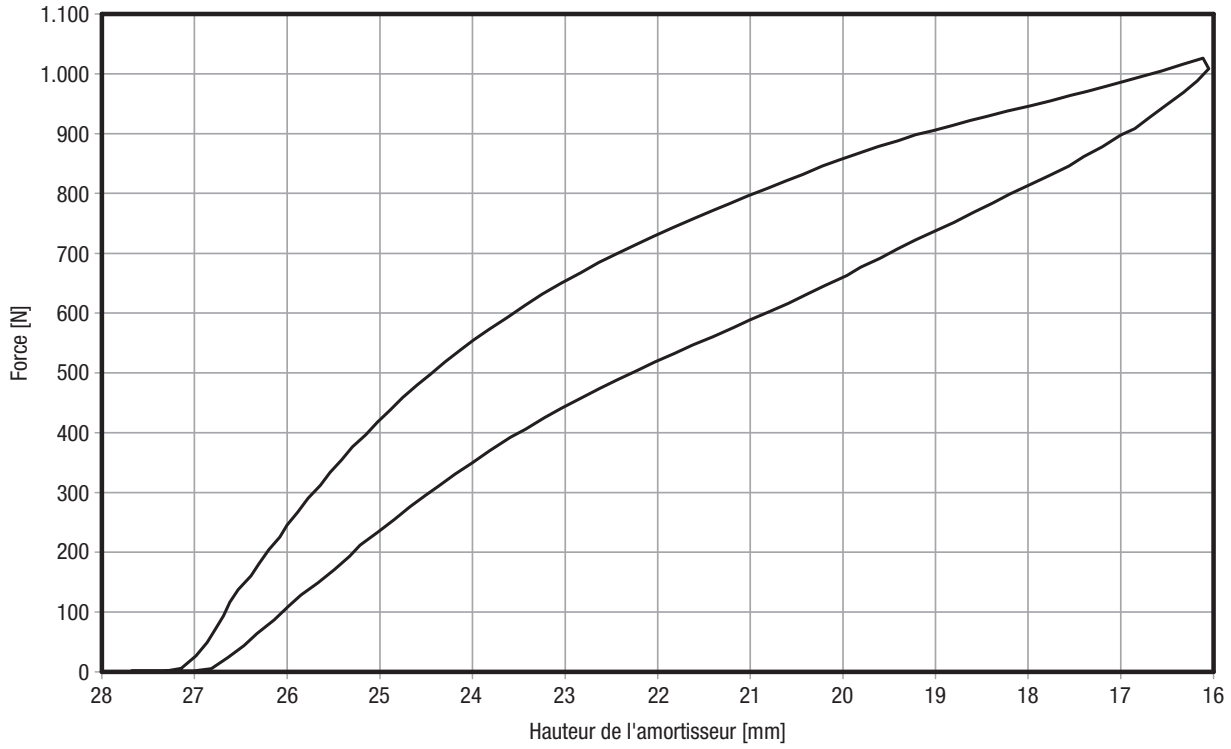
Courbe caractéristique force - course, statique E_{tot} : 7,6 \text{ Nm} , E_{abs} : 1,8 \text{ Nm} , efficacité : 25 %
