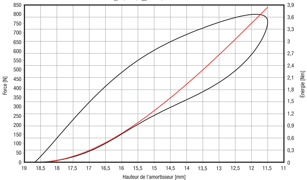
Courbe caractéristique force - course, dynamique E tot : 3,8 Nm, E abs : 2 Nm, efficacité : 53 %
