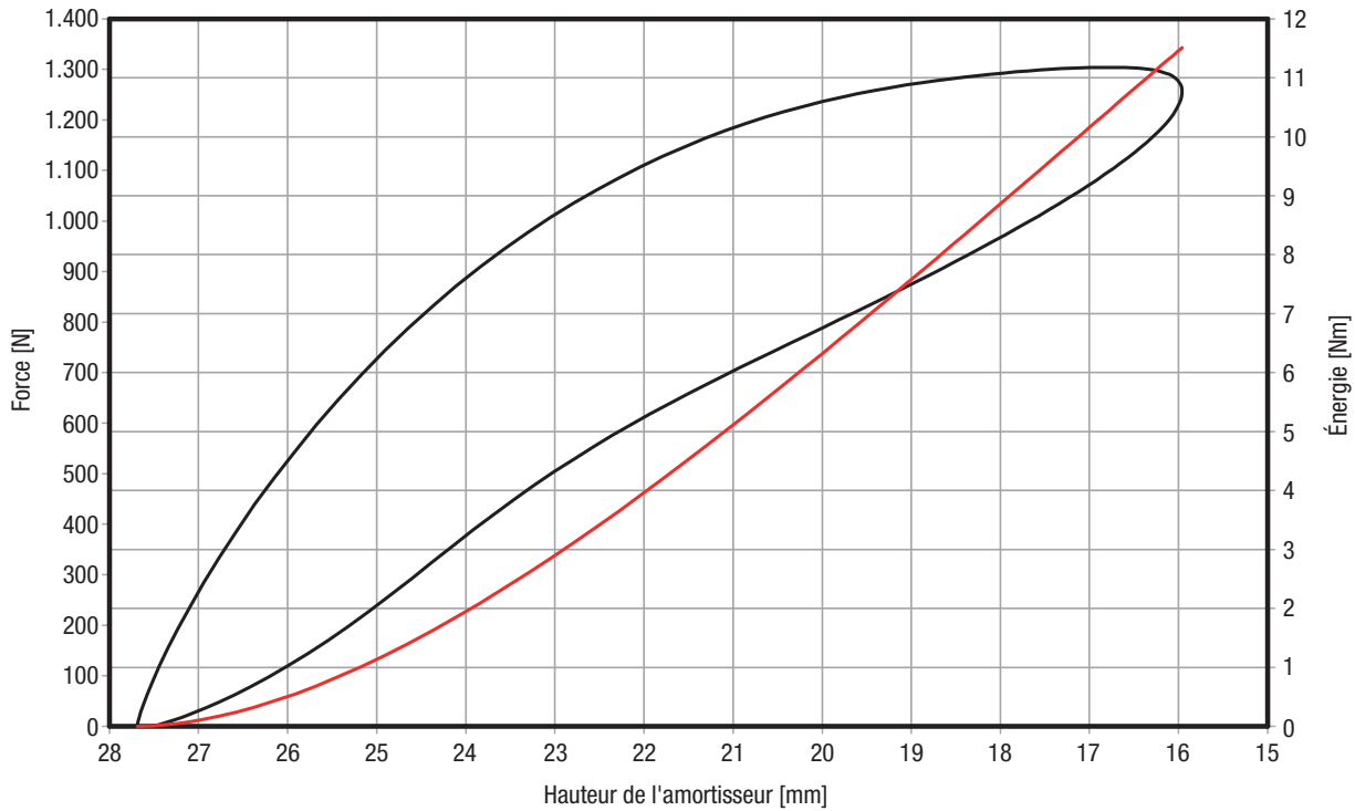
Courbe caractéristique force - course, dynamique E_{tot} : 11,5 \text{ Nm} , E_{abs} : 4,6 \text{ Nm} , efficacité : 40 %
