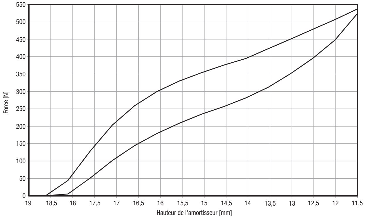
Courbe caractéristique force - course, statique E tot : 2,29 Nm, E abs : 0,65 Nm, efficacité : 28 %
